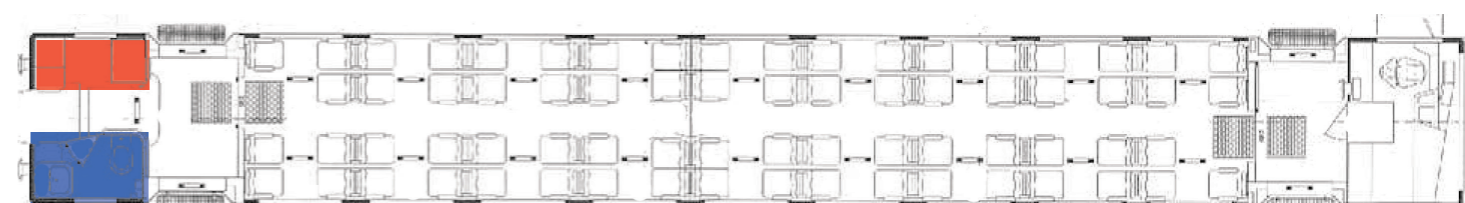
Steuerwagen 2. Klasse (Bt)
