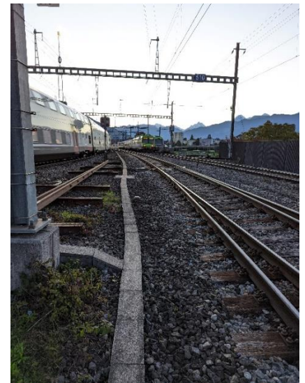
Weiche 412 nahe der Unterführung Simmentalstrasse in Spiez
